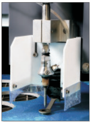
Kollisionsschutz
